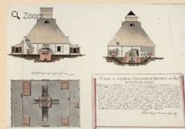
План и профиль стеклянной фабрики в Барнаульском заводе. Чертил бергмейстер 8-го класса П.К. Фролов. [1801 г.] РГИА. Ф. 485. Оп. 5. Д. 841. Л. 13. Подлинник.
